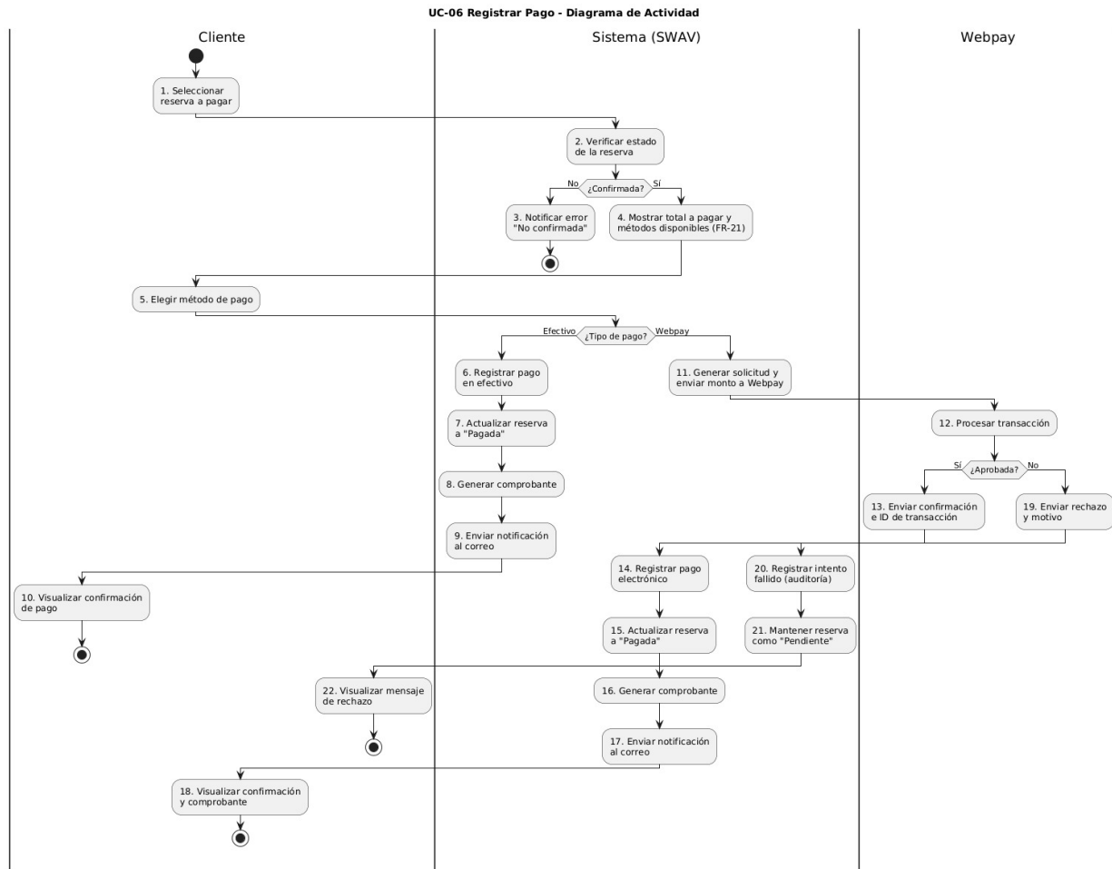
Figura 6: UC-06 – Diagrama de Actividad: Registrar Pago
