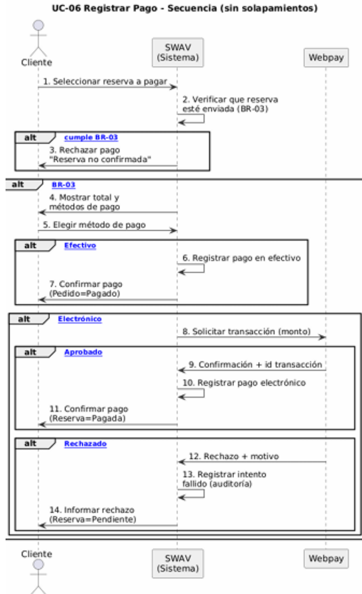
Figura 7: UC-06 – Diagrama de Secuencia: Registrar Pago
