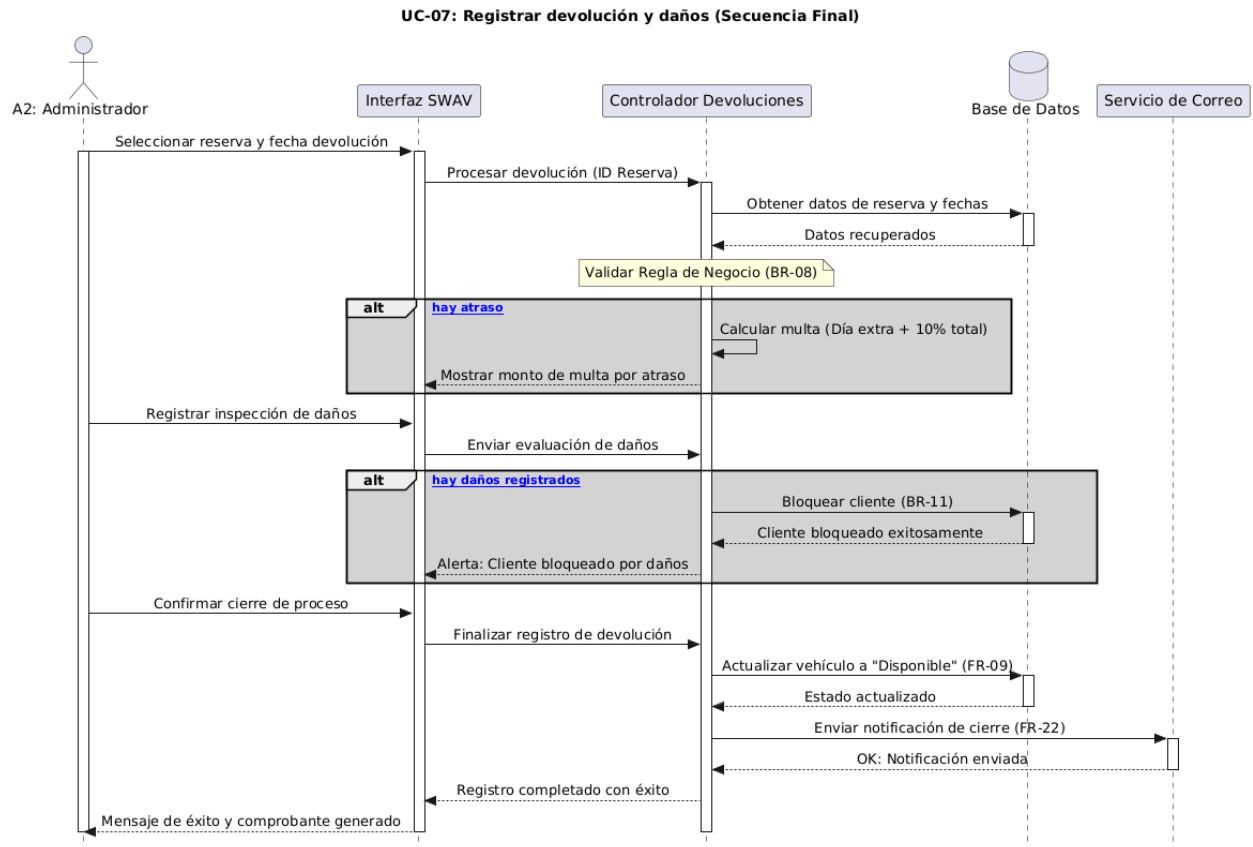
Figura 9: UC-07 – Diagrama de Secuencia: Registrar Devolución y Daños
