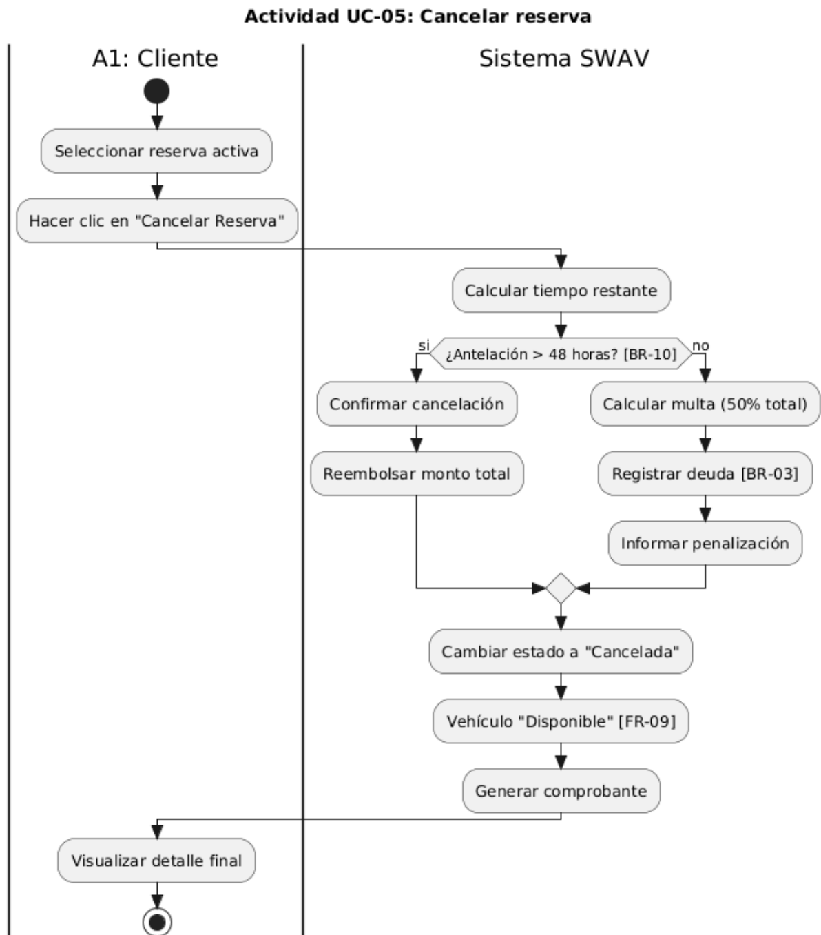
Figura 12: UC-05 – Diagrama de Actividad: Cancelar Reserva
