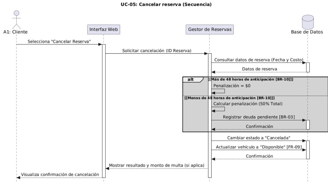
Figura 13: UC-05 – Diagrama de Secuencia: Cancelar Reserva
