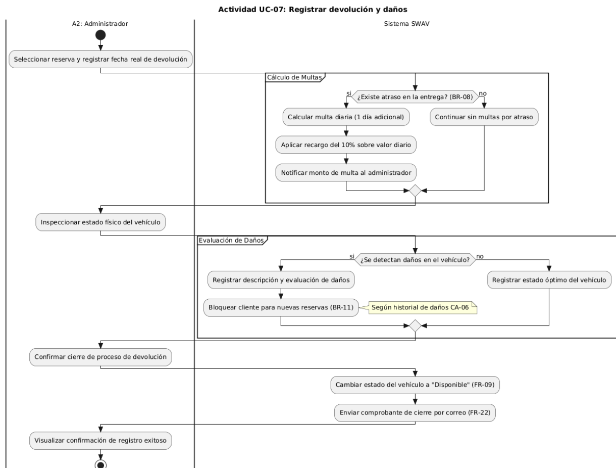
Figura 8: UC-07 – Diagrama de Actividad: Registrar Devolución y Daños
