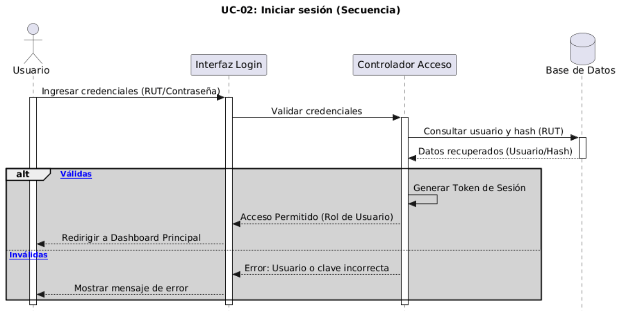
Figura 10: UC-02 – Diagrama de Secuencia: Iniciar Sesión
