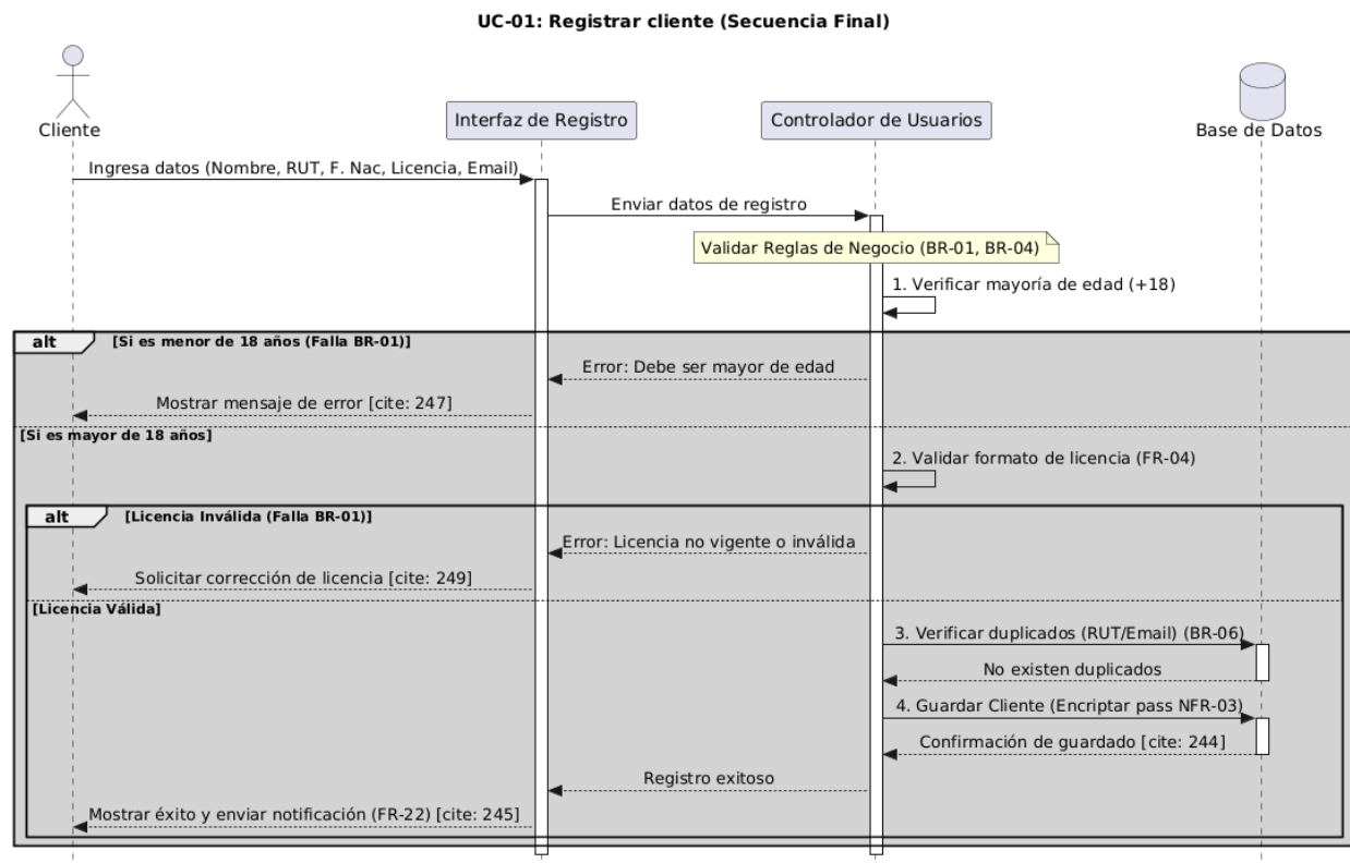
Figura 4: UC-01 – Diagrama de Secuencia: Registrar Cliente
