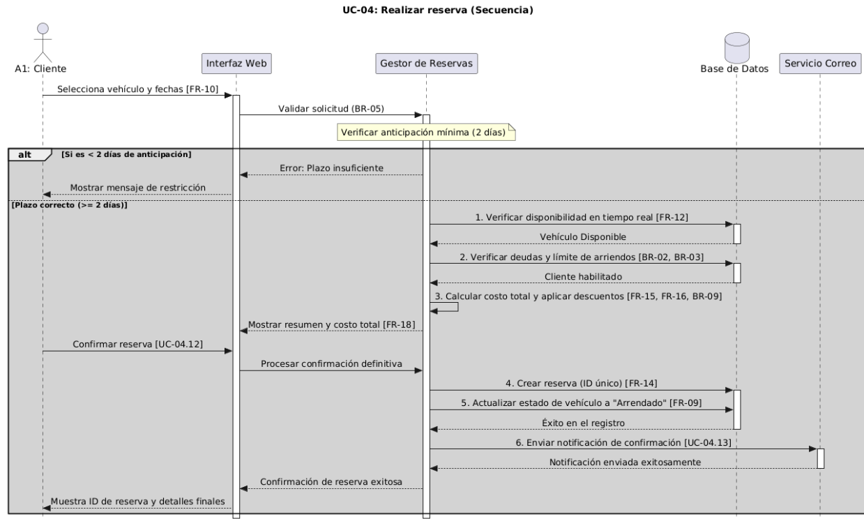
Figura 5: UC-04 – Diagrama de Secuencia: Realizar Reserva
