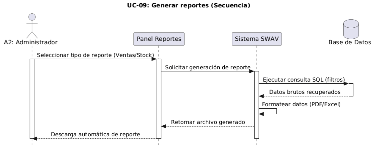
Figura 15: UC-09 – Diagrama de Secuencia: Generar Reportes
