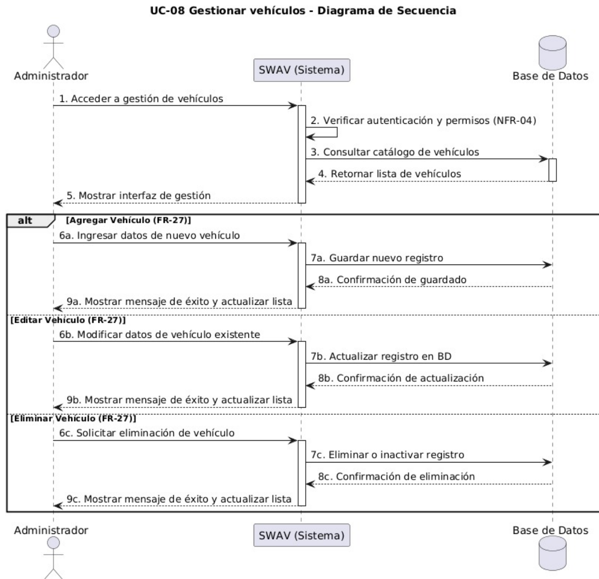
Figura 14: UC-08 – Diagrama de Secuencia: Gestionar Vehículos
