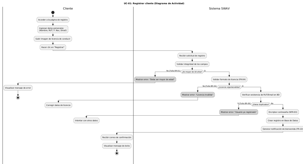
Figura 3: UC-01 – Diagrama de Actividad: Registrar Cliente
