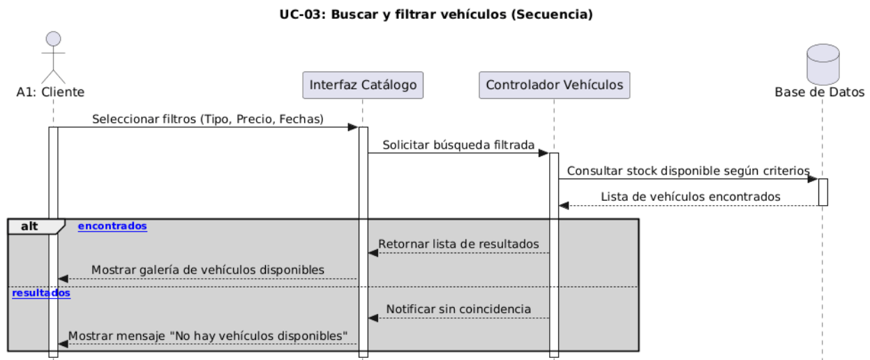
Figura 11: UC-03 – Diagrama de Secuencia: Buscar y Filtrar Vehículos
