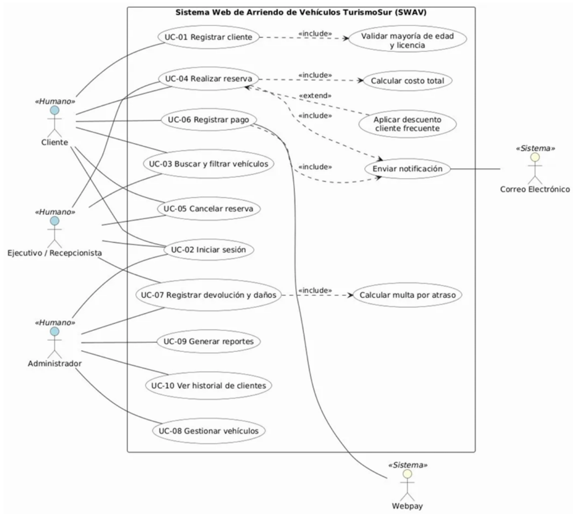
Figura 2: SWAV – Diagrama de Casos de Uso
