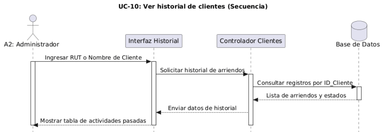
Figura 16: UC-10 – Diagrama de Secuencia: Ver Historial de Clientes
